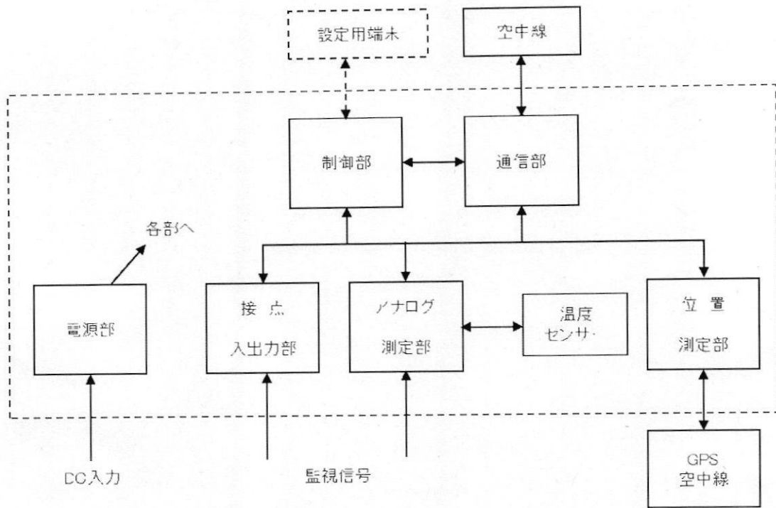
第1図 系統図
