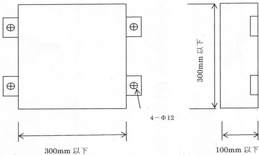
第2図 概観図
