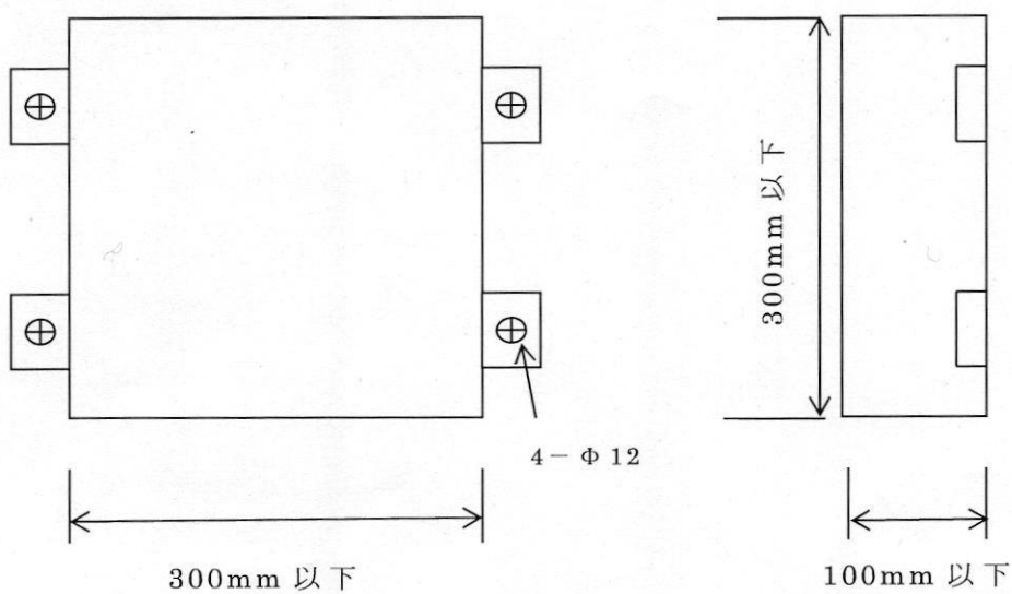
第 2 図 概観図
