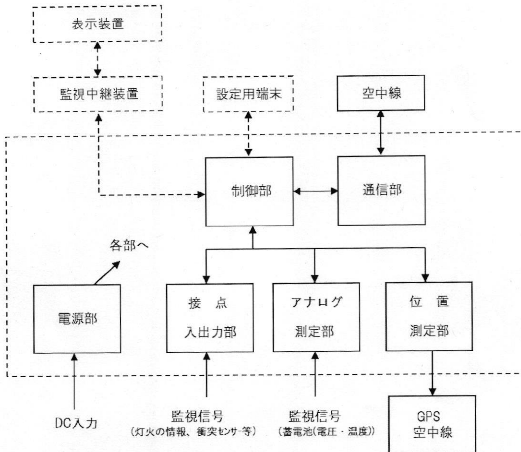
第 1 図 系統図
