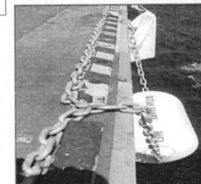
移設する防舷物の設置状況
