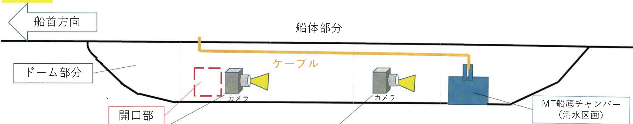
MT船底チャンバー (清水区画) の図面
