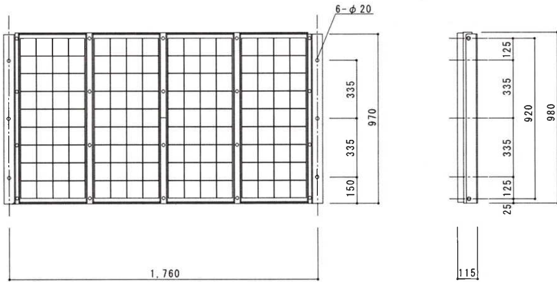
太陽電池架 外形寸法図
