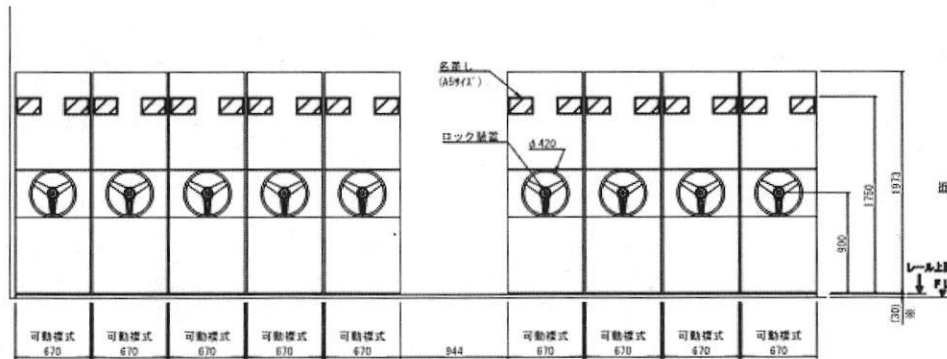
姿図 S=1/40
