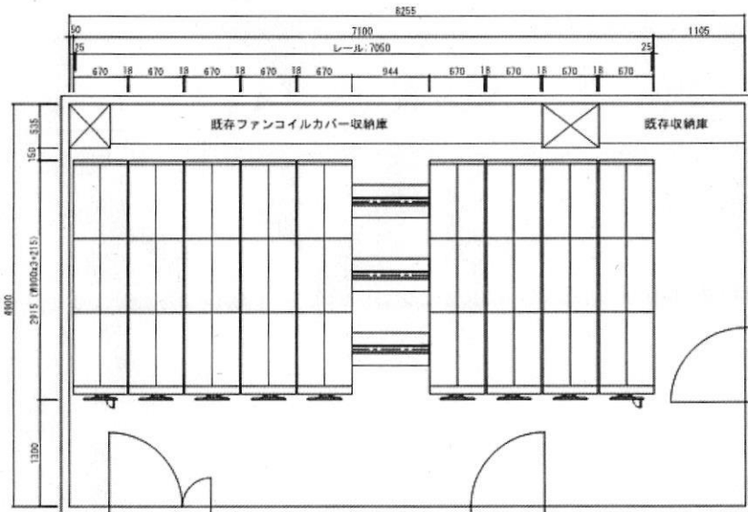
配置図 S=1/50
