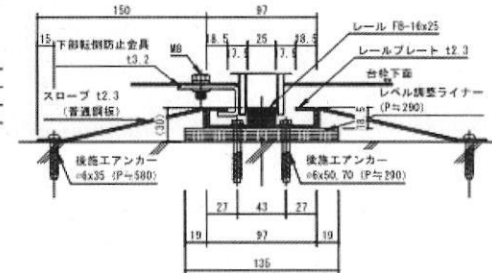
据置レール (スロープ付) 詳細図 S=1/4
