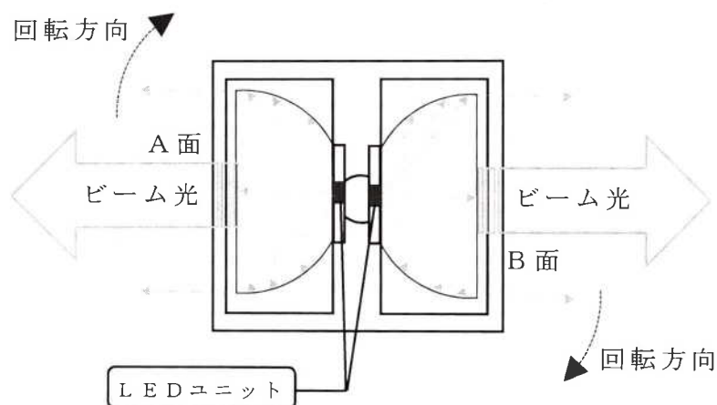
図 2. 灯体内部を上面から見た一例
