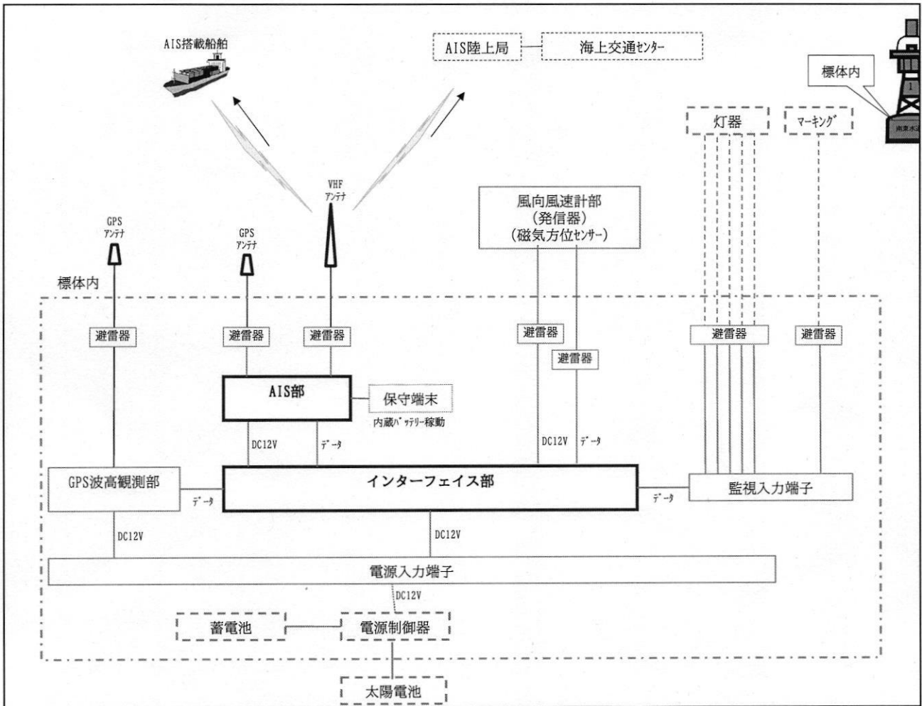
灯浮標用気象観測装置系統図
