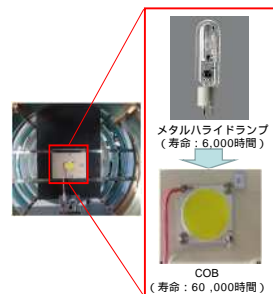
COB (寿命：60,000時間)
